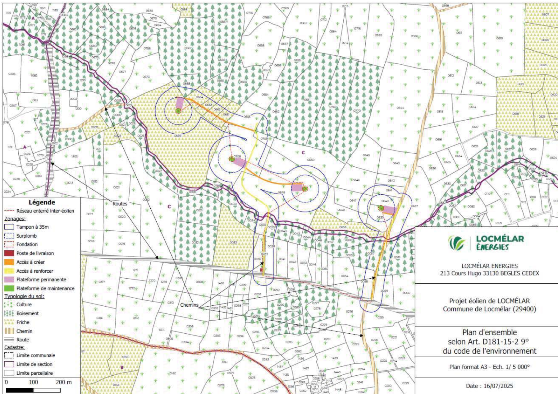
Figure 23 : Plan de masse du projet (Source : VALOREM)
