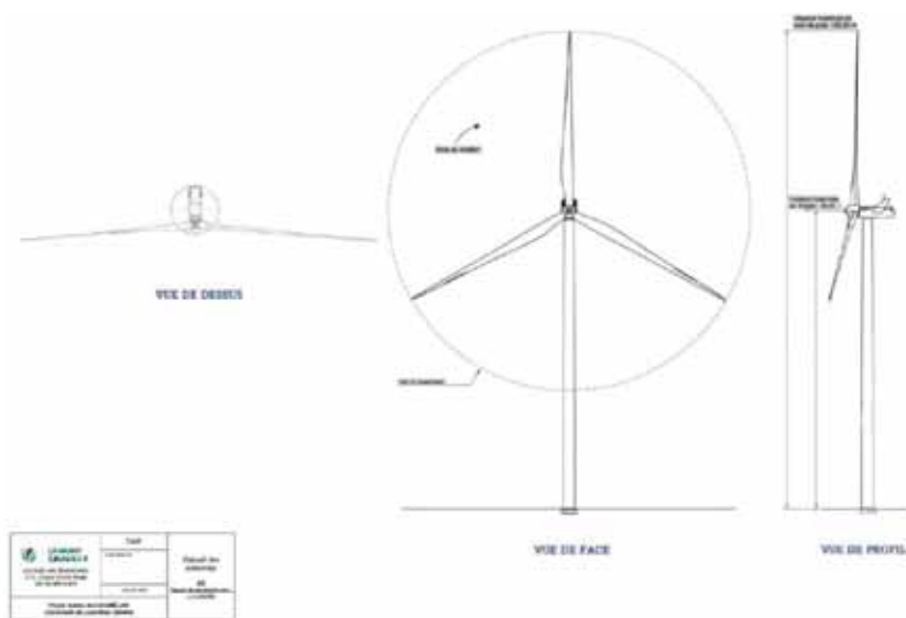
Figure 24 : Gabarit maximum de l'éolienne retenue (VALOREM)
